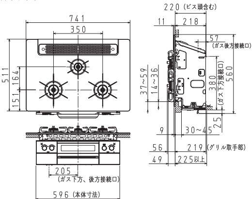
本図面はPD-893WS-75GH
