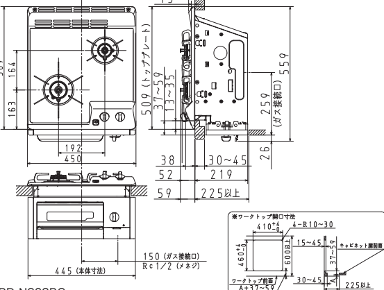
本図面はPD-N202BG
